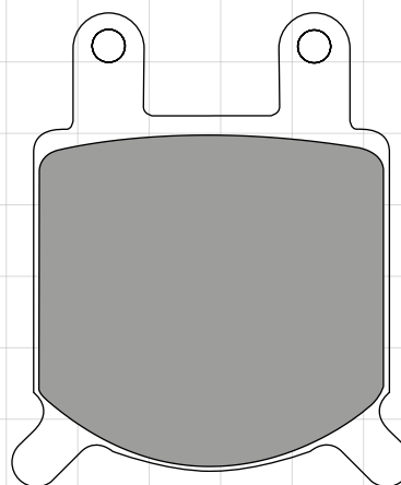
DP917 49 x 58 x 7.1mm
