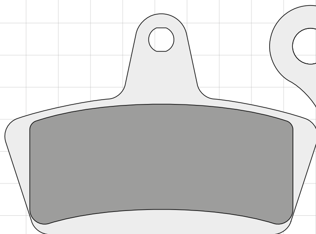
DP530 84.4 x 59.7 x 10.1mm
